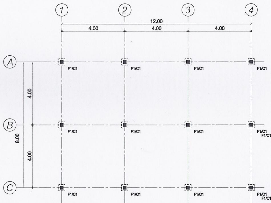
แปลนฐานราก
