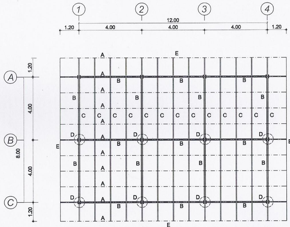
แปลนโครงหลังคา
