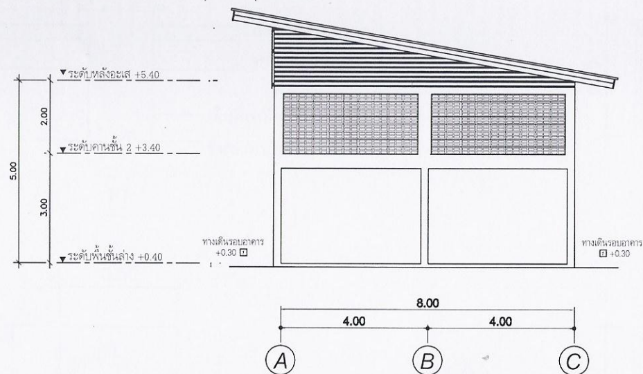
รูปด้าน 4 SCALE 1:100
