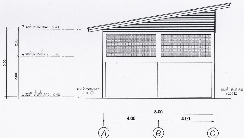
รูปด้าน 2
